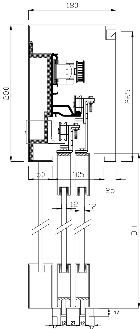
단면도
